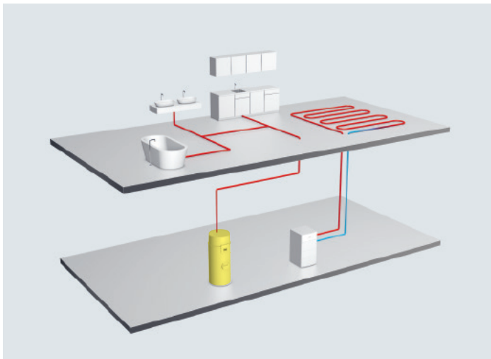
Schematische Darstellung von Raumheizung und Warmwasseraufbereitung bei einem Einfamilienhaus mit dem Wärmepumpenboiler Oertli TWH Pro und einer Öl- oder Gasheizung.
